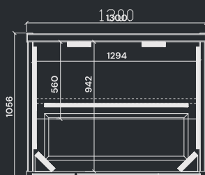
Ansicht 1
