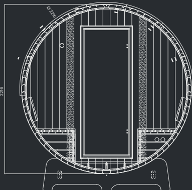
Frontansicht
