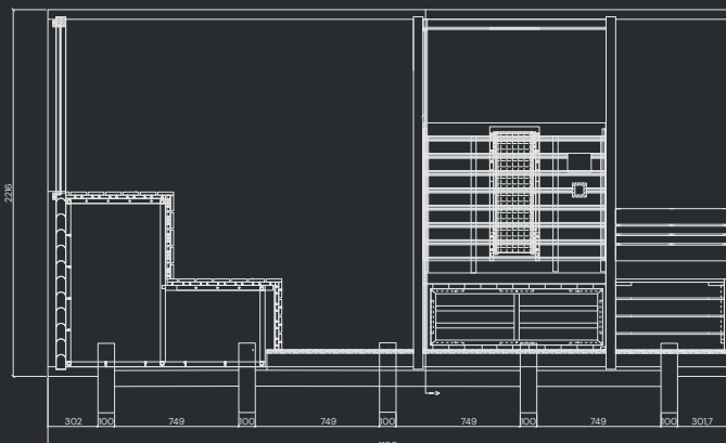
Seitenansicht
