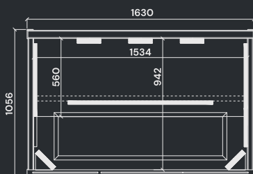
Ansicht 1
