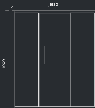
Ansicht 2
